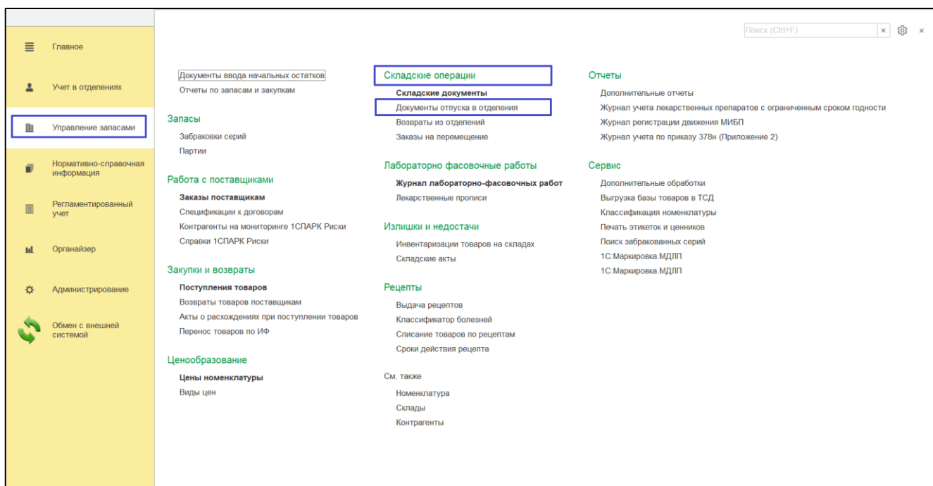
Рисунок 68 – Начальная страница
