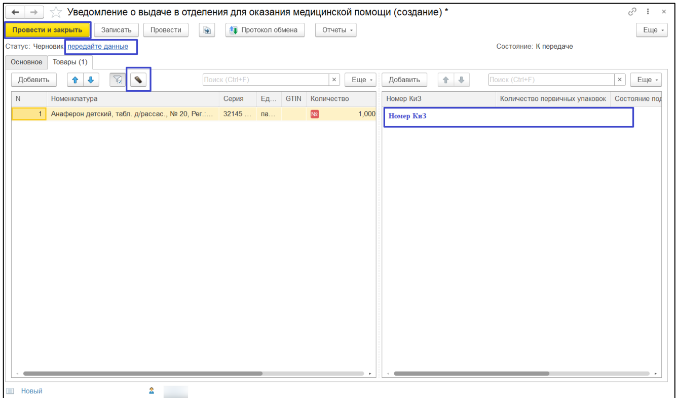
Рисунок 72 – Вкладка "Товары"
