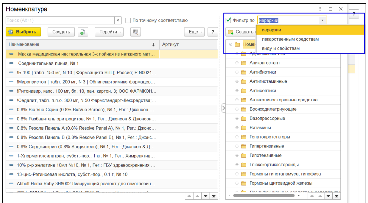
Рисунок 34 – Панель фильтров
