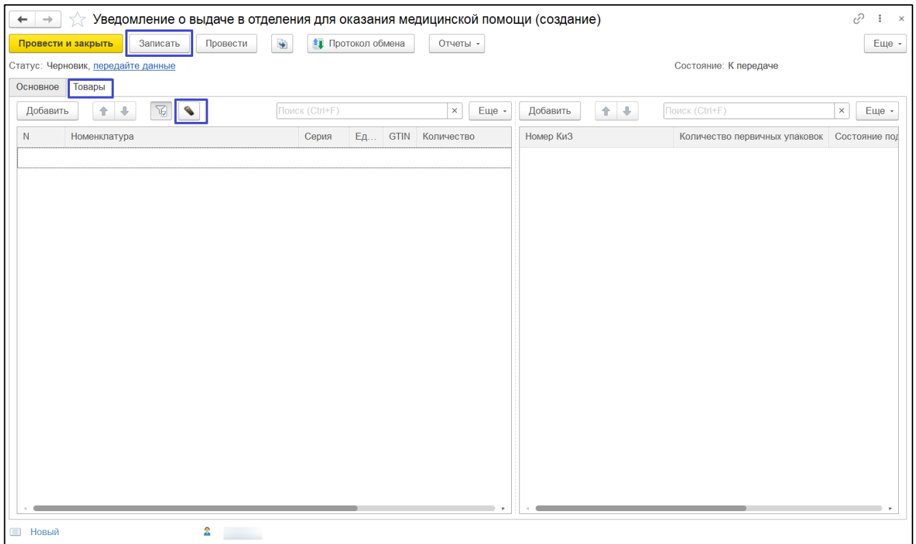
Рисунок 78 – Вкладка "Товары"
