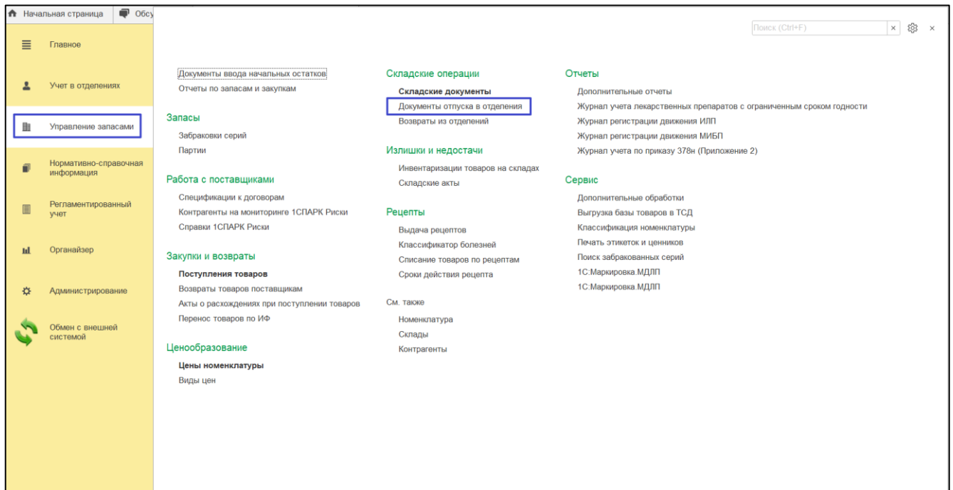
Рисунок 95 – Начальная страница
