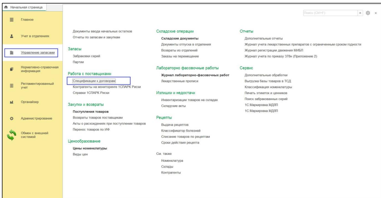
Рисунок 45 – Начальная страница
