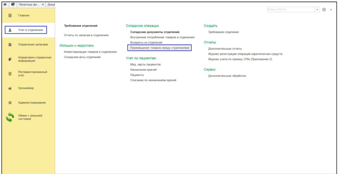
Рисунок 100 – Начальная страница
