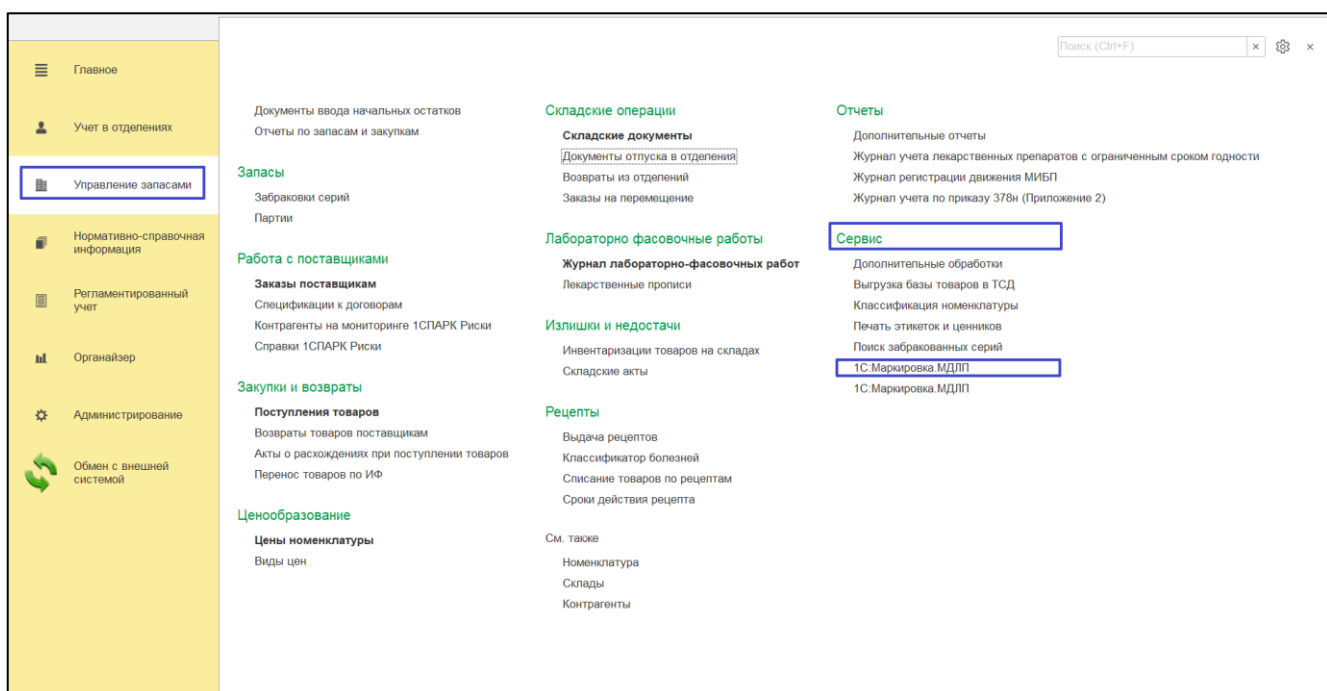
Рисунок 74 – Начальная страница
