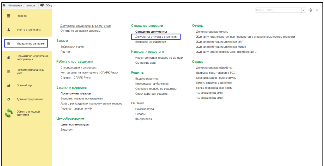
Рисунок 83 – Начальная страница
