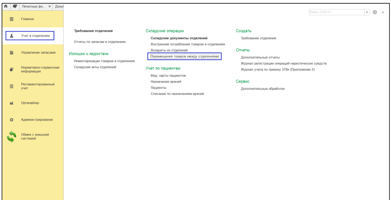
Рисунок 88 – Начальная страница
