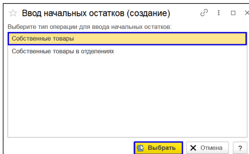
Рисунок 108 – Кнопка "Выбрать"
