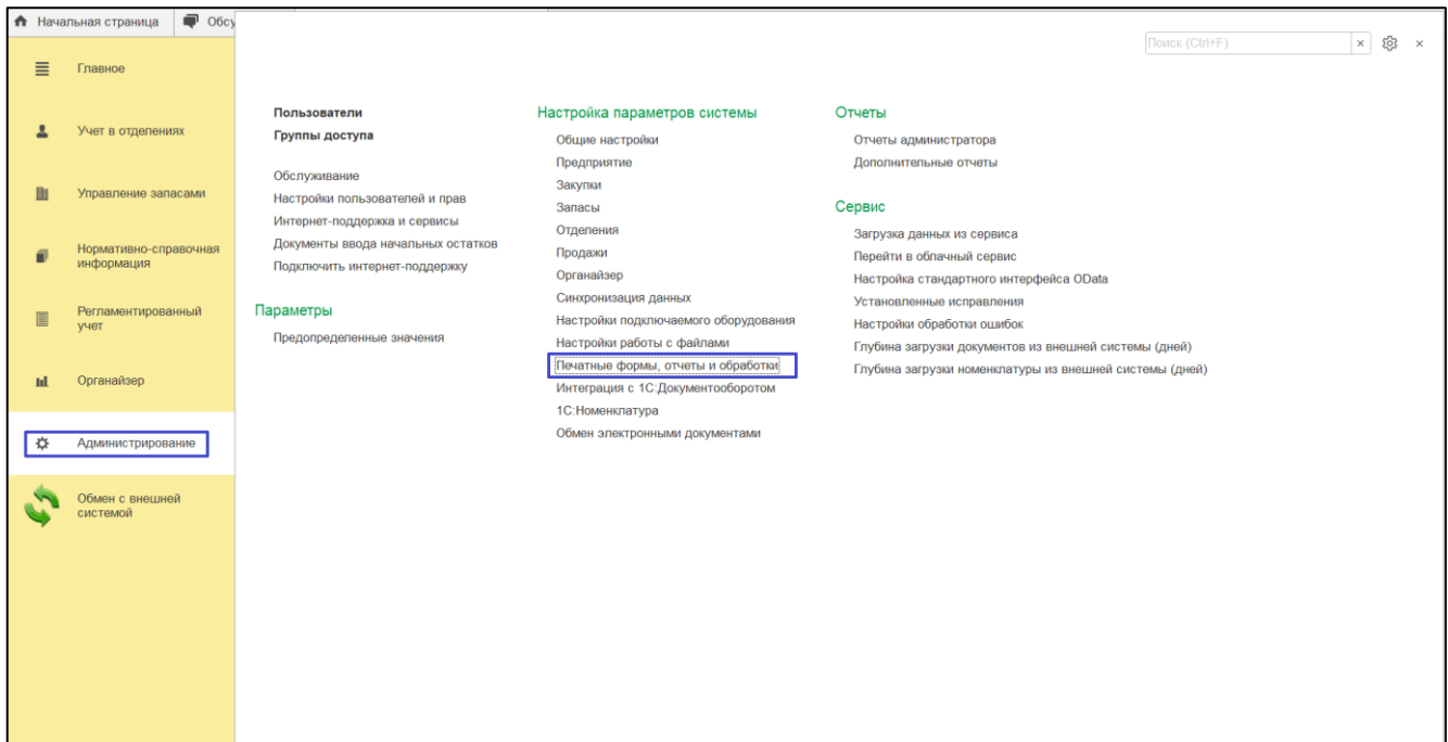
Рисунок 93 – Начальная страница
