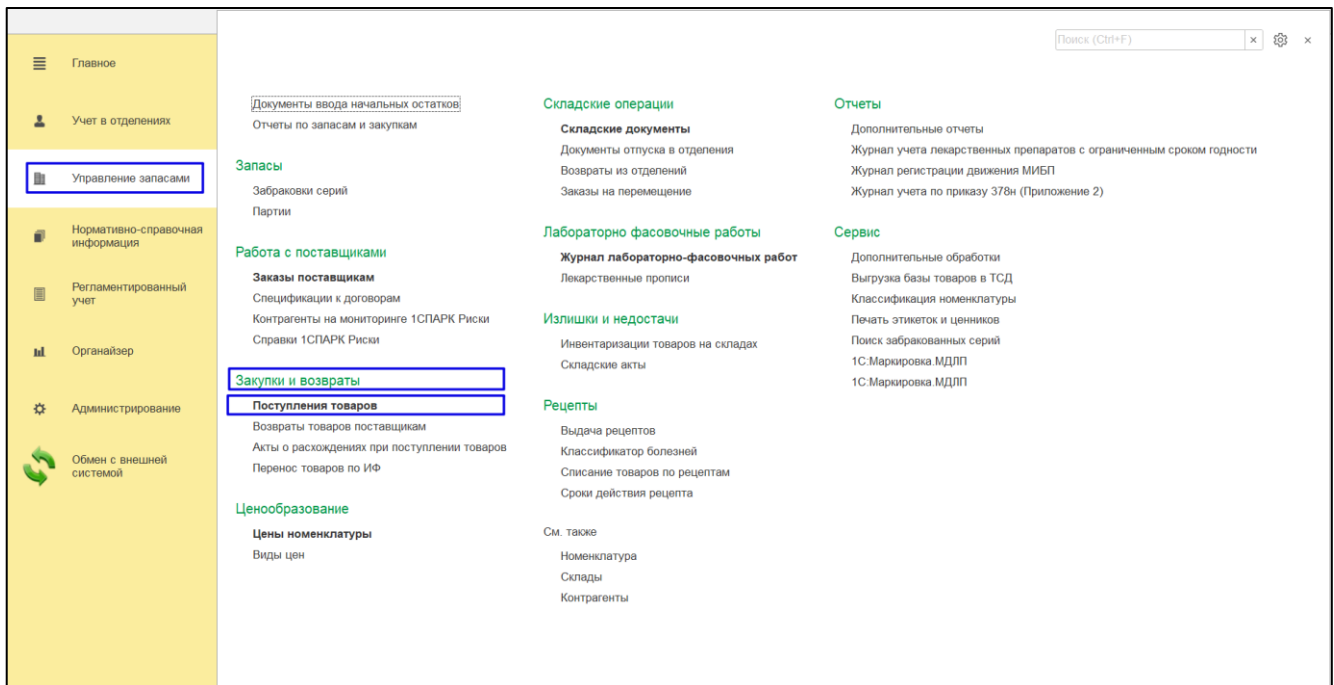
Рисунок 6 – Начальная страница
