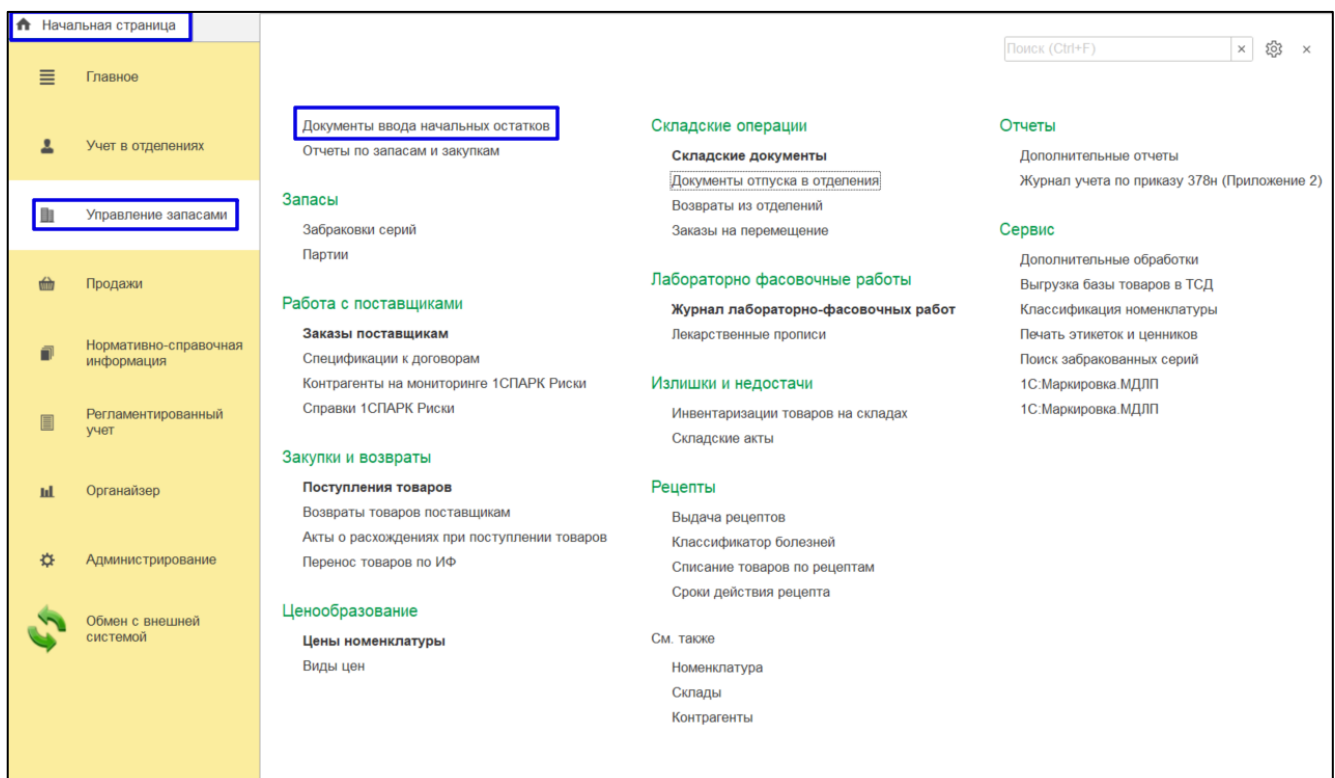
Рисунок 105 – Начальная страница
