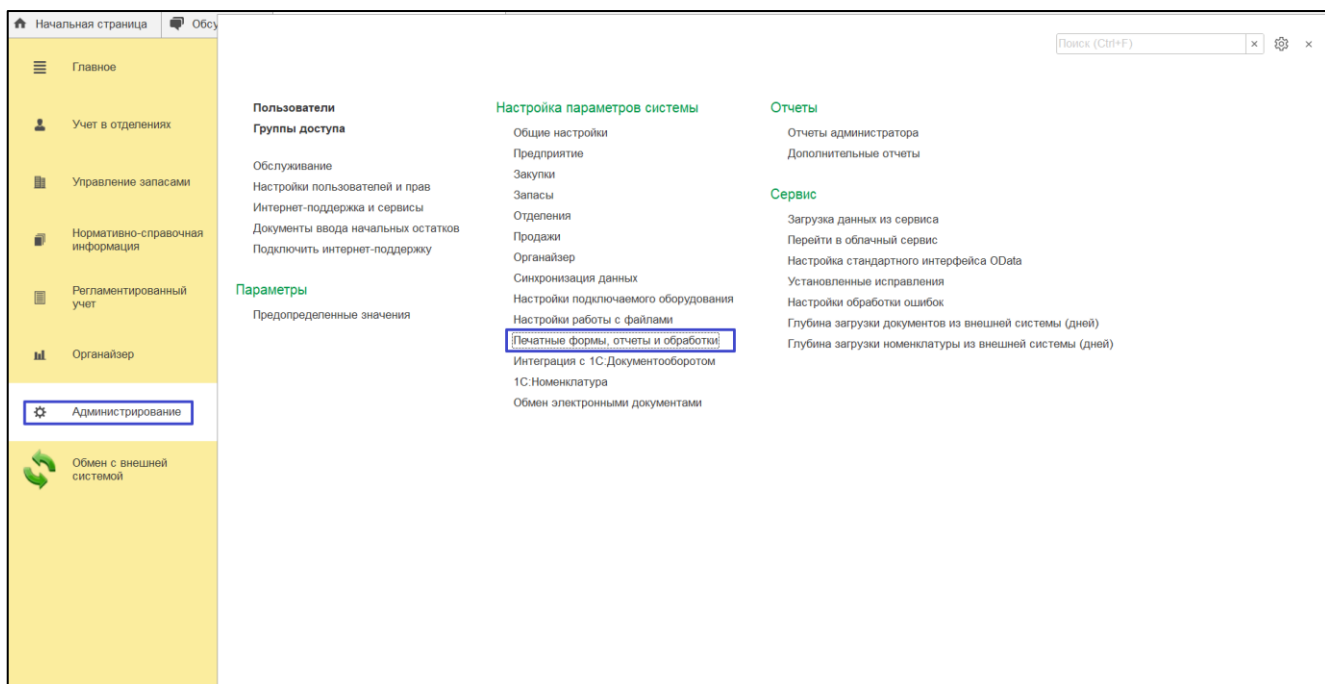
Рисунок 81 – Начальная страница
